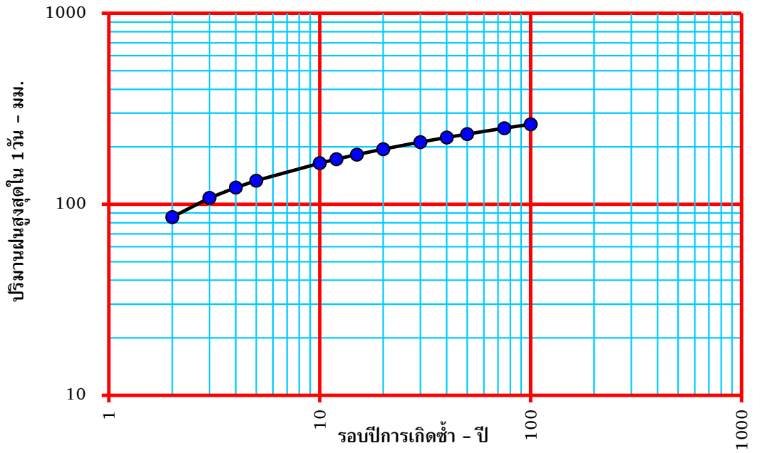
แสดงรอบปีการเกิดซ้ำปริมาณฝนสูงสุดใน 1 วัน สถานี วัดไกลกังวล ต.หัวหิน อ.หัวหิน จ.ประจวบคีรีขันธ์
