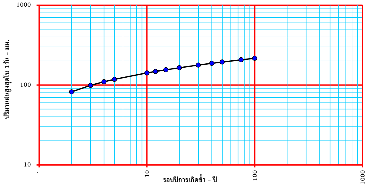
แสดงรอบปีการเกิดซ้ำปริมาณฝนสูงสุดใน 1 วัน สถานี 450231 (Gt.9) คลองทับสะแก อ.ทับสะแก จ.ประจวบคีรีขันธ์
