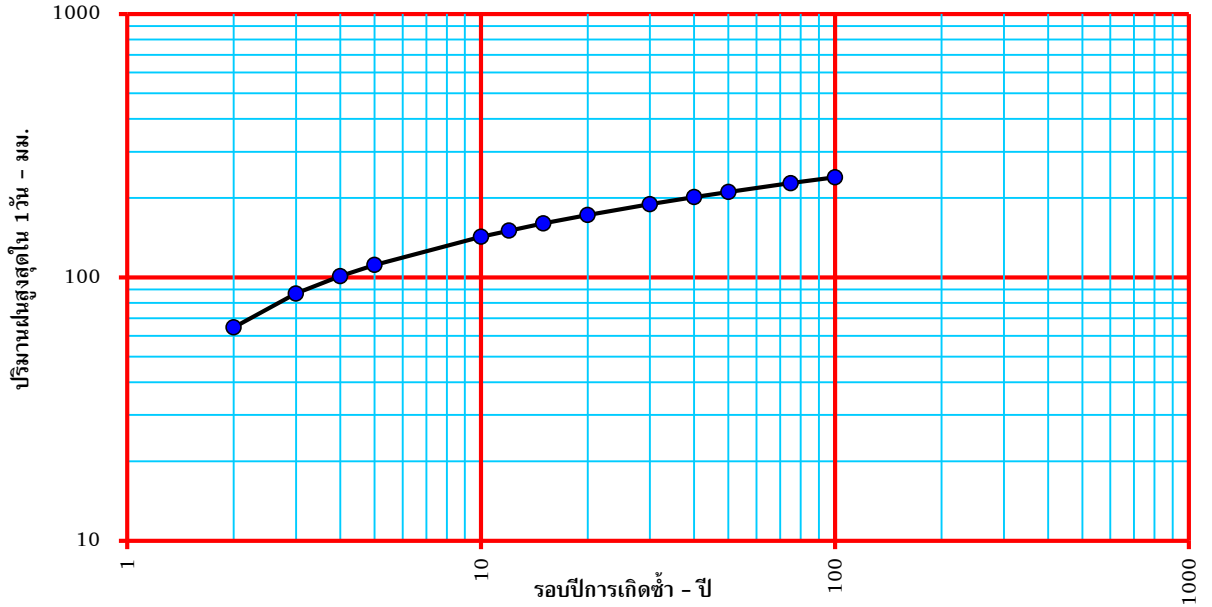
แสดงรอบปีการเกิดซ้ำปริมาณฝนสูงสุดใน 1 วัน สถานี 370560 (B.8A) อ.ท่าช้าง จ.เพชรบุรี
